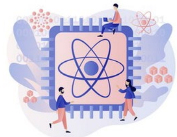
Computación Cuántica
